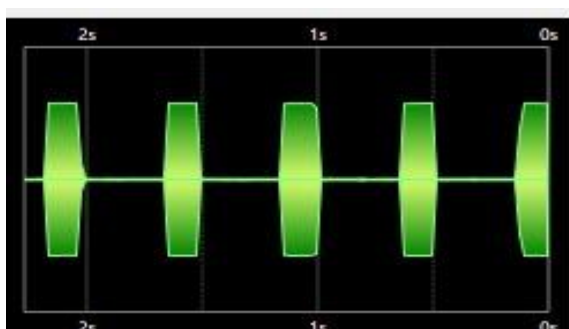
Génération de la modulation OOK avec fronts « anti-claquements »
