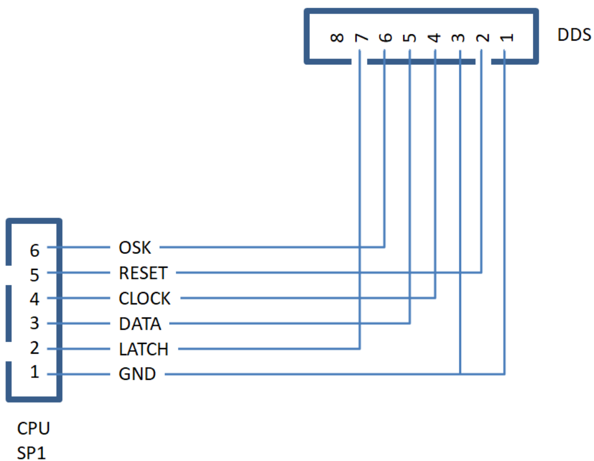
Câble FbBalise vers connecteur DDS
